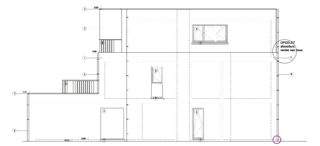
ZIJGEVEL LINKS
