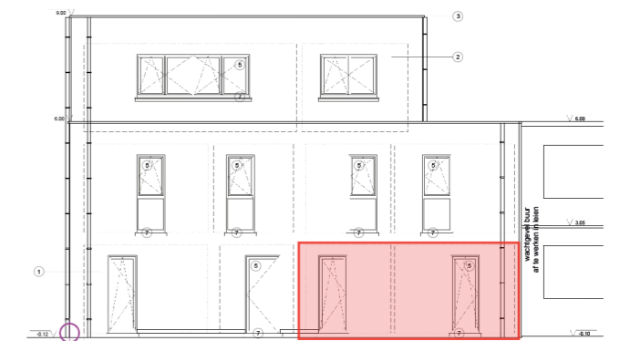
VOORGEVEL
