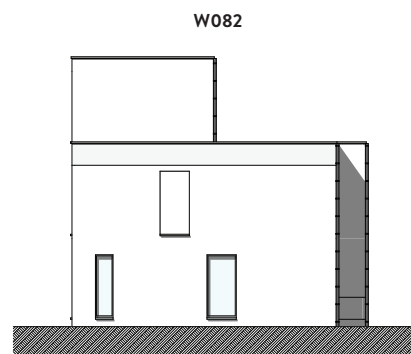
RECHTERGEVEL
