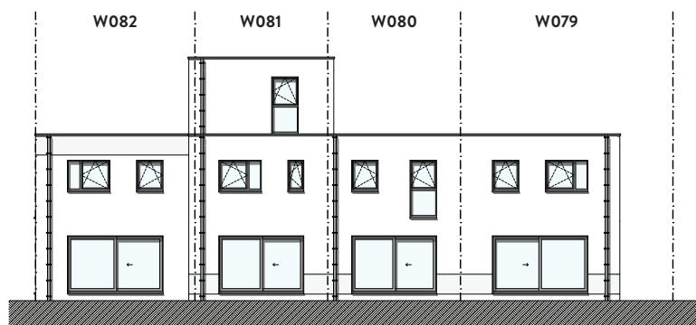
ACHTERGEVEL
